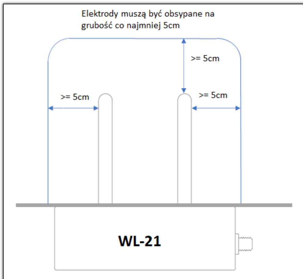
Rysunek 2 Zasypanie elektrod czujnika materiałem
