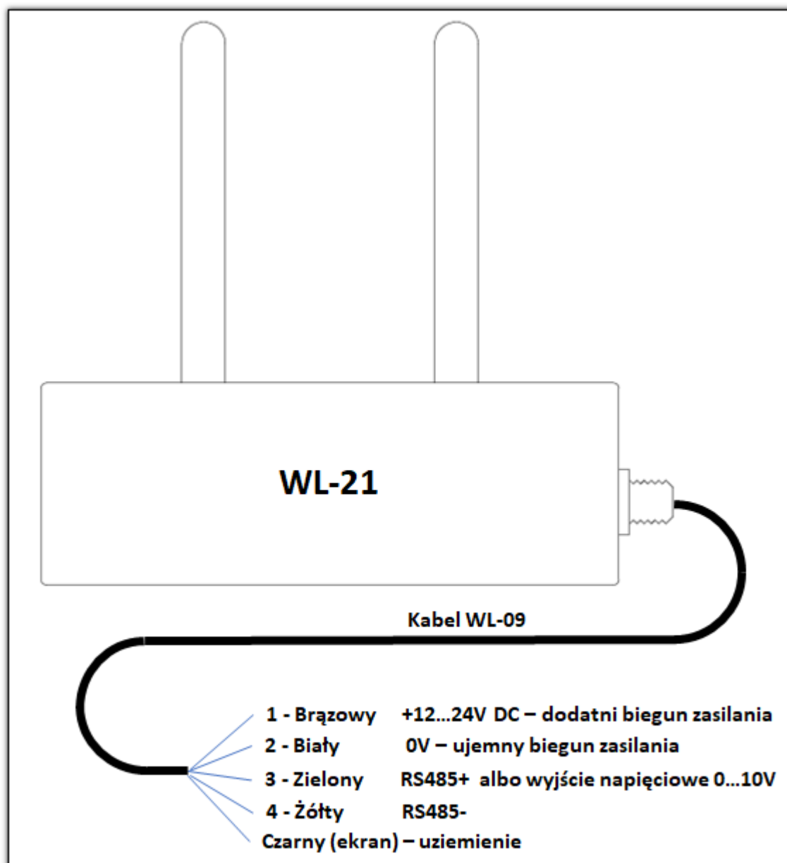
Rysunek 4 Podłączenie elektryczne czujnika
