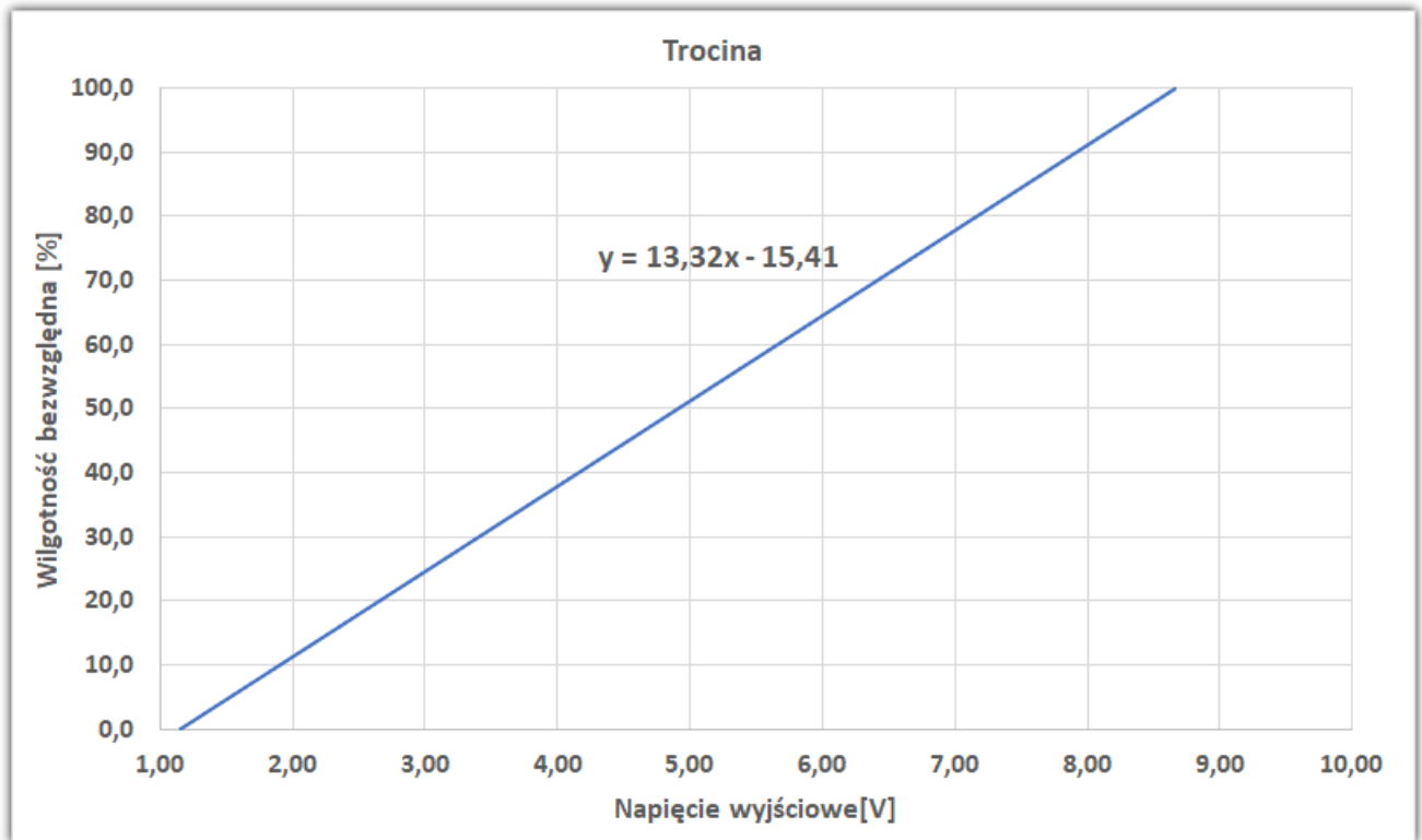
Rysunek 5 Przykładowa charakterystyka wyjściowa czujnika dla trocin
