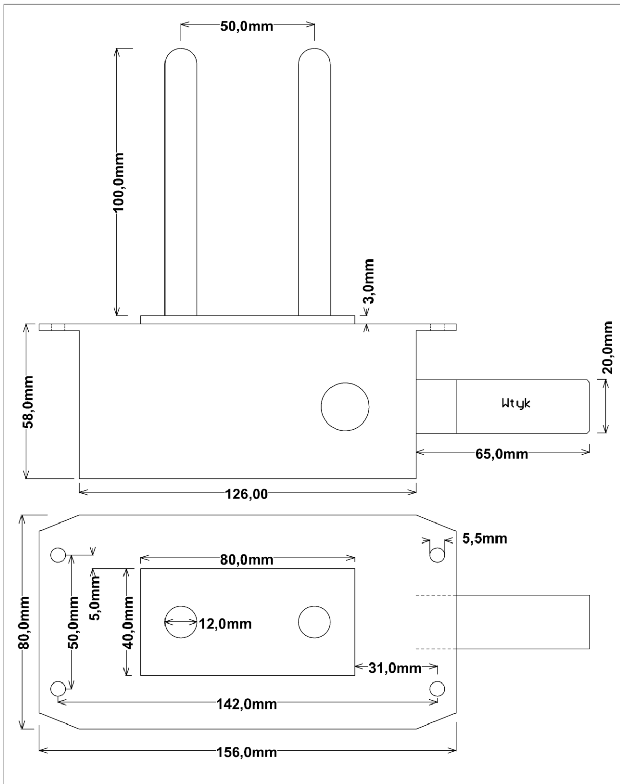
Rysunek 5 Wymiary czujnika
