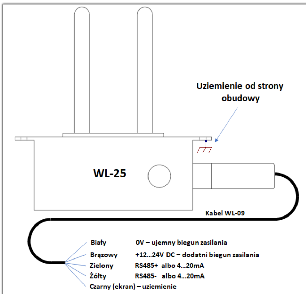
Rysunek 3 Podłączenie elektryczne czujnika
