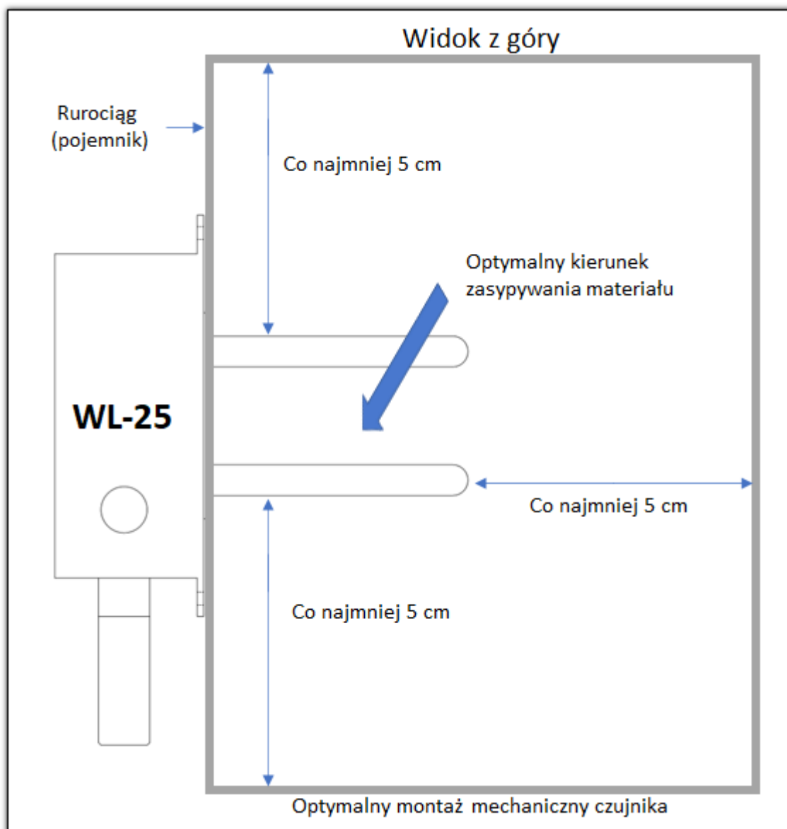
Rysunek 1 Montaż mechaniczny czujnika
