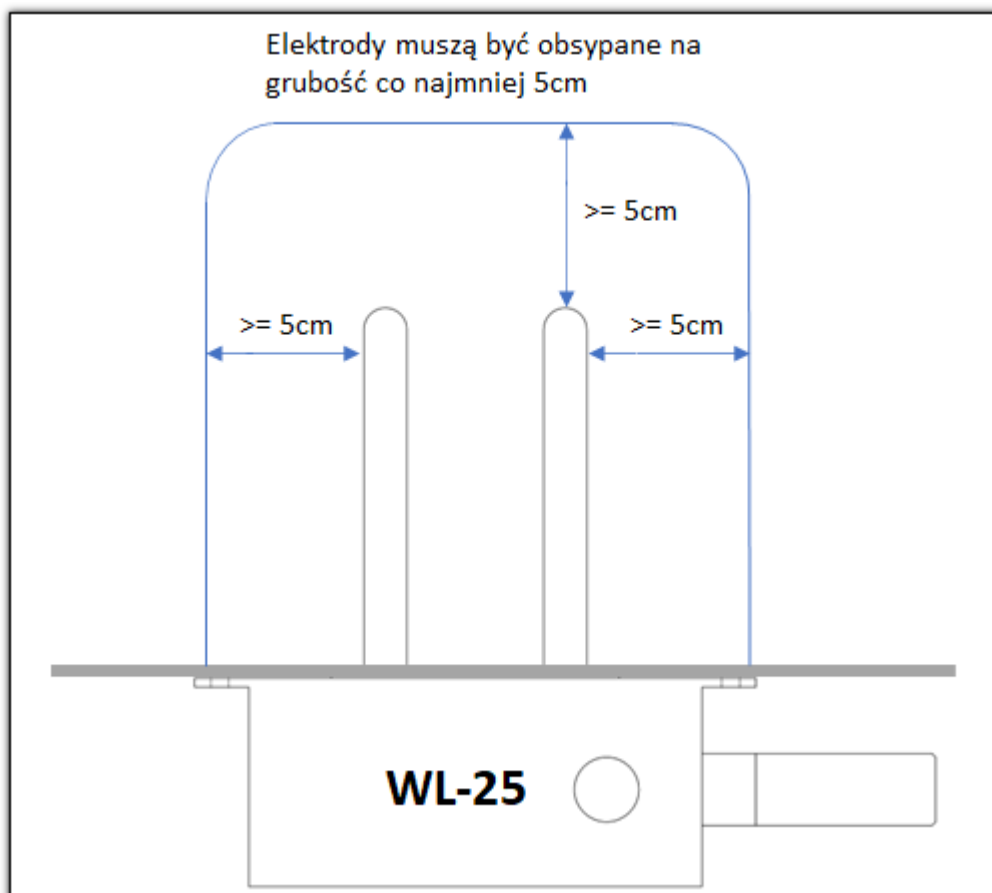
Rysunek 2 Zasypanie elektrod czujnika materiałem
