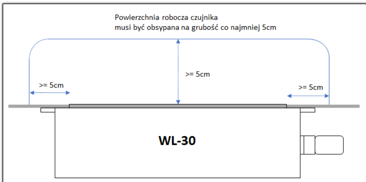
Rysunek 2 Zasypanie czujnika materiałem
